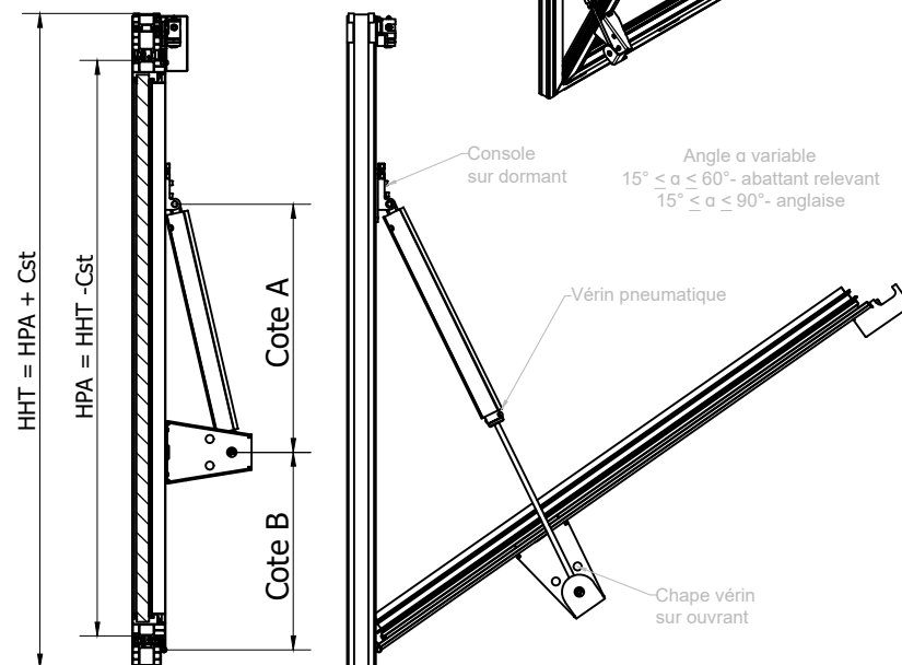
A-A ( 1:10 )
